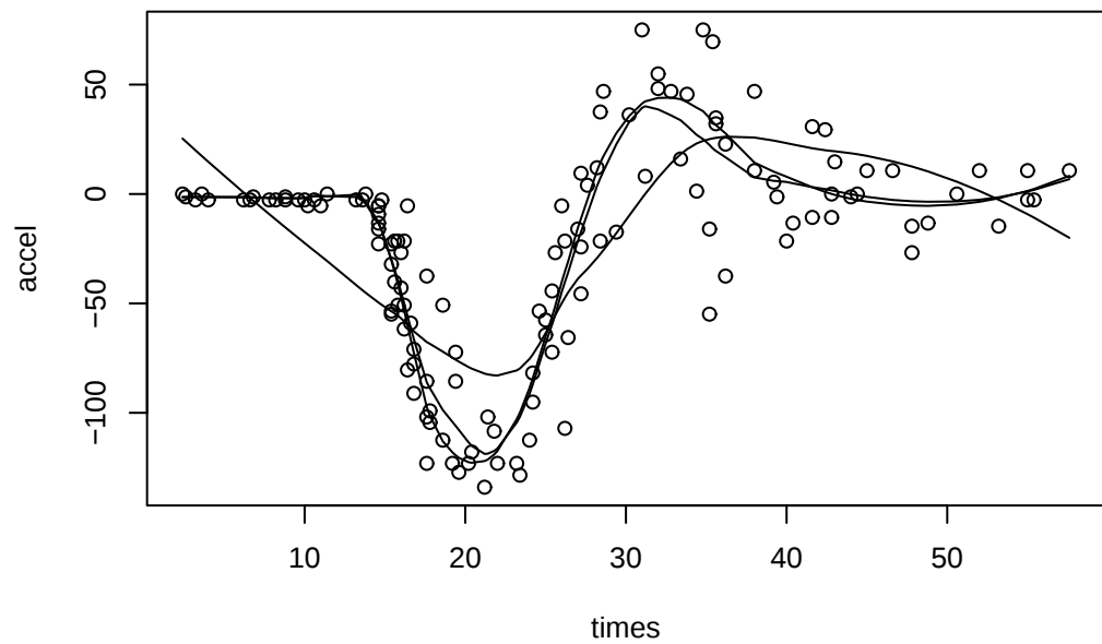
Loess
