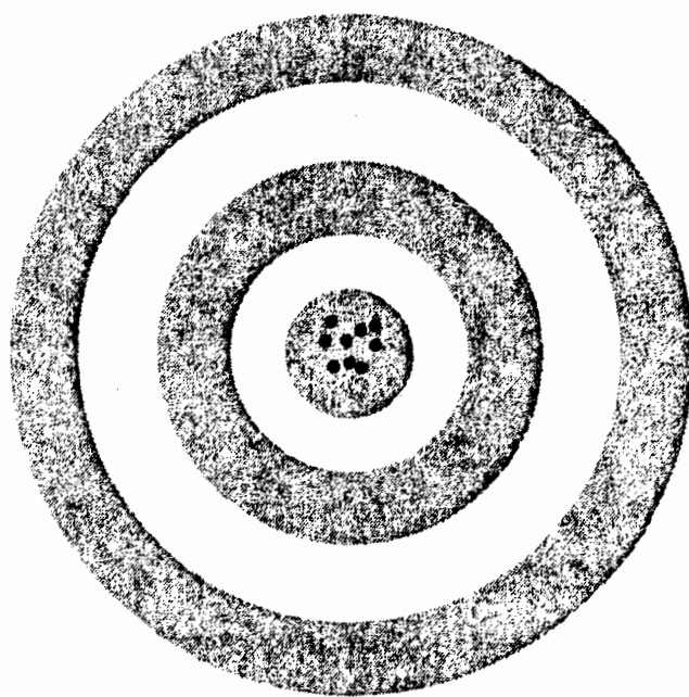
(d) Low bias, high precision
