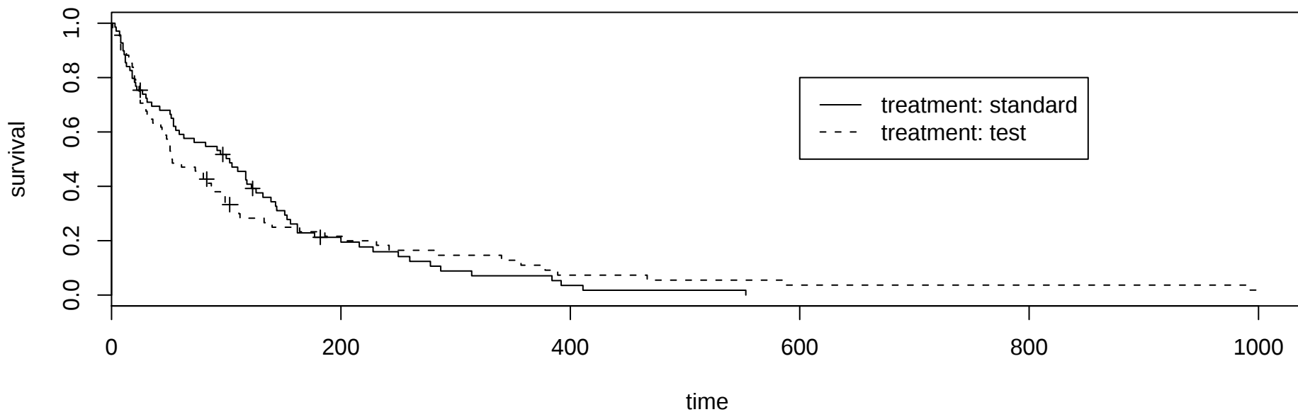
Kaplan-Meier estimators (VA data)
